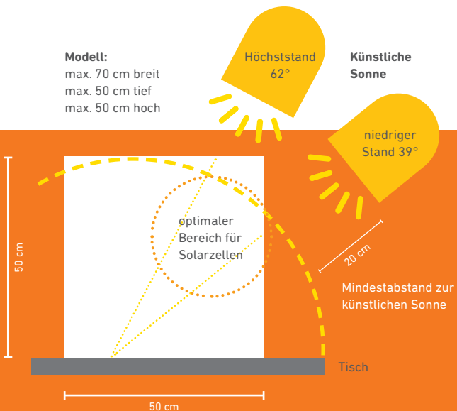
Die Solarteststation in Seitenansicht
